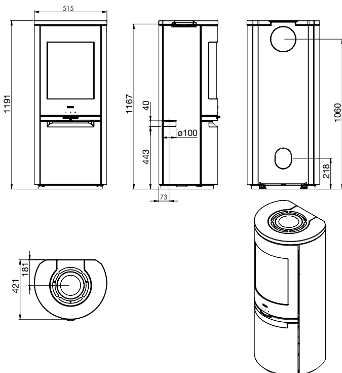
Scan-Line 900 Serie
